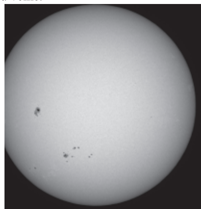
Sluneční skvrny na povrchu Slunce
