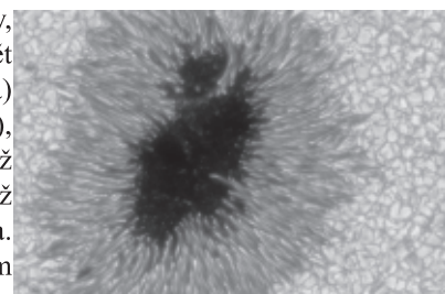
Sluneční skvrna "zblízka"
