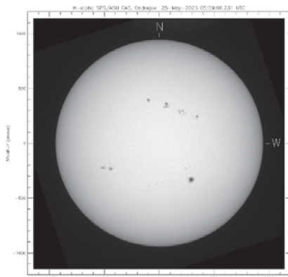
Slunce se slunečními skvrnami zachycené Sluneční patrolou (Sluneční oddělení, Astronomický ústav AV ČR) 25. května 2023
