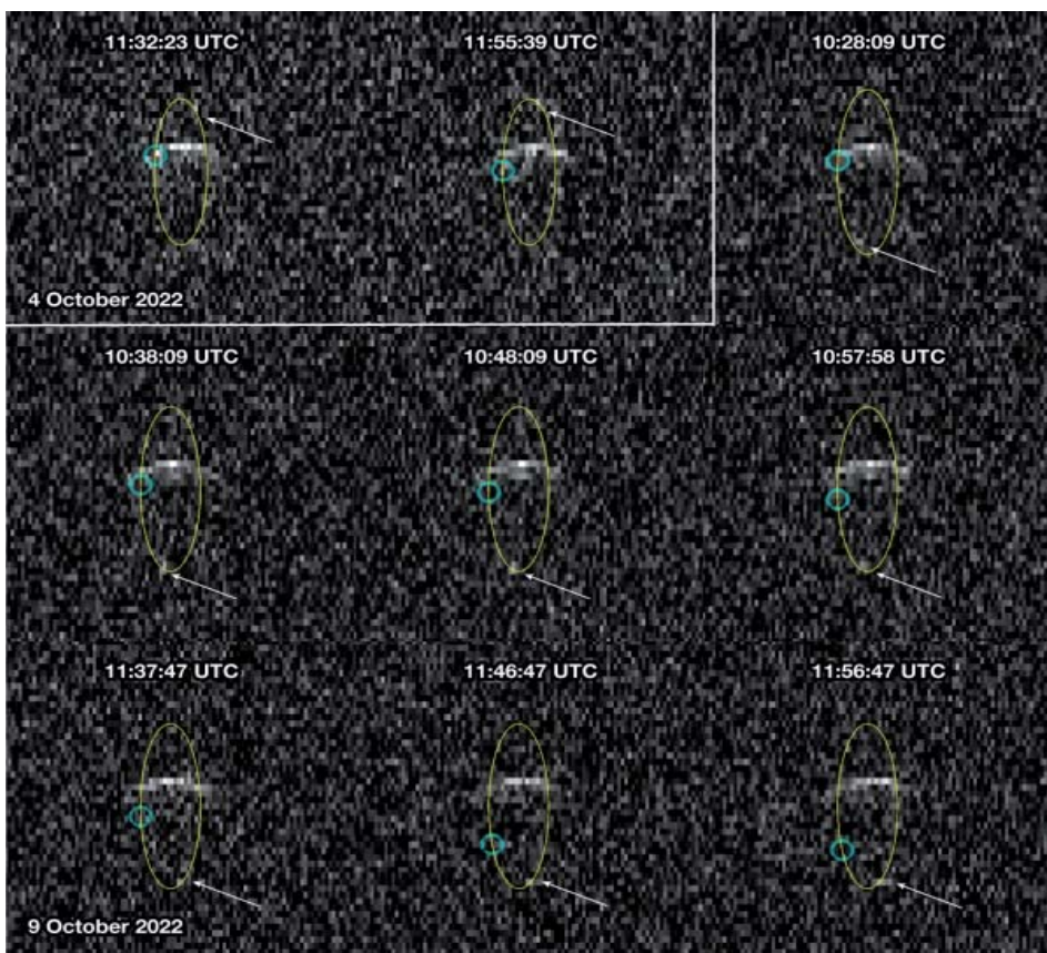
Sekvence radarových snímků pořízených 4. října 2022 (výřez) a 9. října 2022. Zobrazen je odraz od hlavního tělesa – Didyma – a také od menšího Dimorphos. Pro zvýraznění je průmět modelové dráhy překreslen žlutou elipsou a šipka ukazuje k místu, kde se Dimorphos nachází. Modrá kružnice pak ukazuje pozici, kde by se měsíček měl nacházet, kdyby nedošlo ke srážce se sondou DART.
